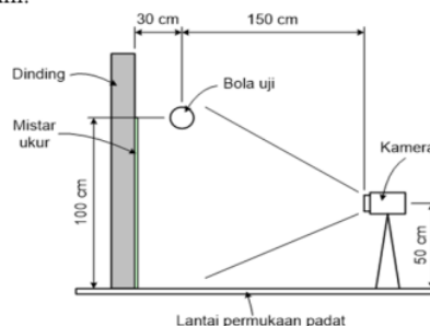
Gambar 1. Skema pengambilan data (Irwanto et al., 2021).
