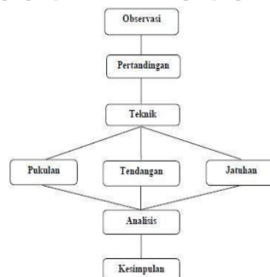
Gambar 1. Desain Penelitian
