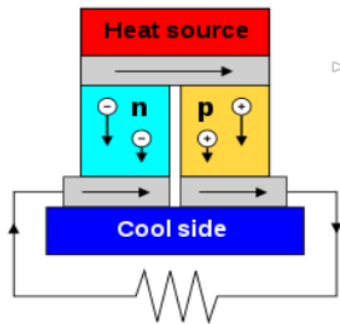
Gambar 1. prinsip kerja generator termoelektrik
