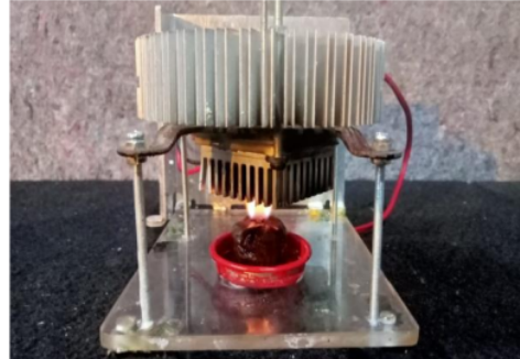
Gambar 2. Rangkaian alat generator termoelektrik
