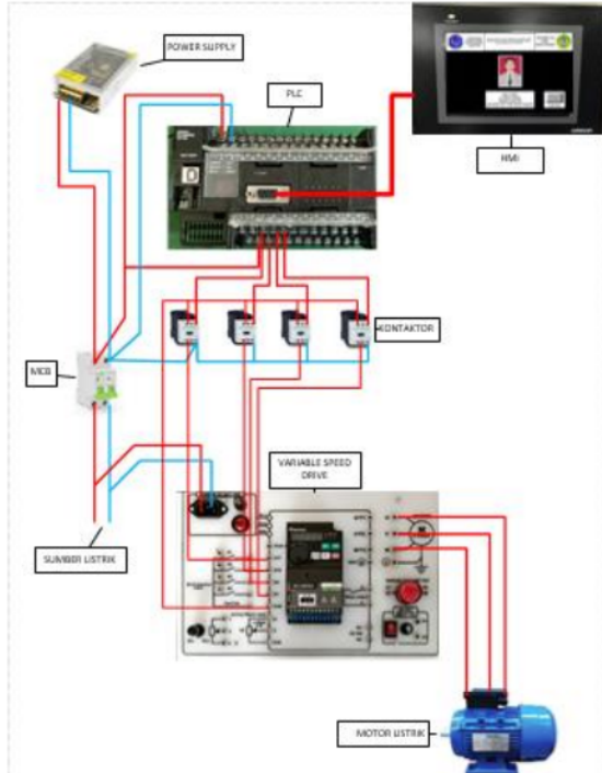
Gambar 2. Desain Sistem Kontrol
