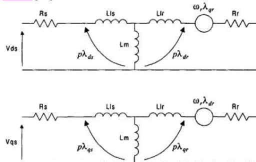
Gambar 2. Rangkaian Ekuivalen Motor Induksi [10]
