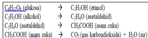
Gambar 1. Persamaan Reaksi
