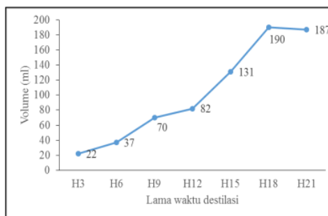
Gambar 5. Hasil Proses Destilasi
