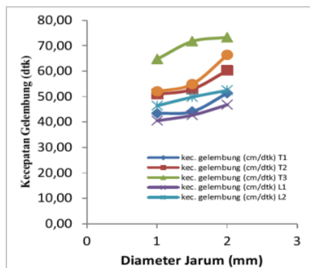
Gambar 2. grafik kecepatan gelembung terhadap diameter jarum
