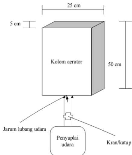
Gambar. 1 Rancang bangun kolom aerator
