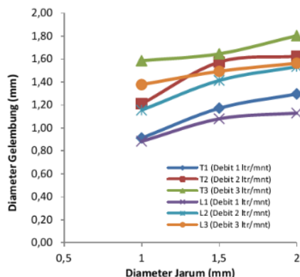
Gambar 2. Grafik rata – rata diameter gelembung.
