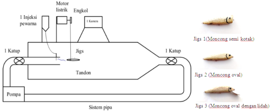
Gambar 1. Skema alat penelitian
