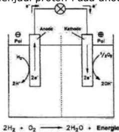
Gambar 1. Skema kerja fuel cell
