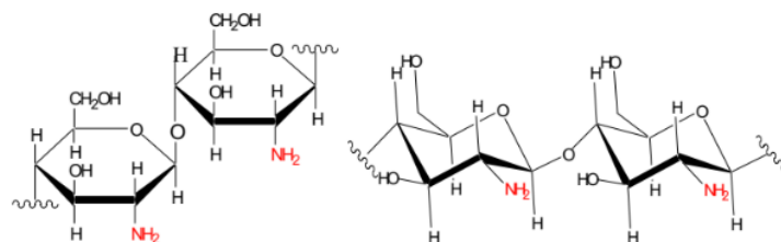
Gambar 3. Struktur kimia kitosan
