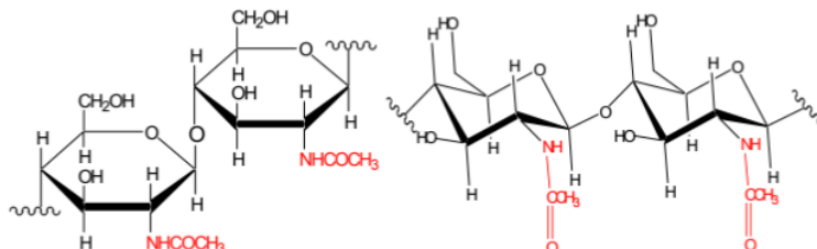
Gambar. 2 struktur kitin
