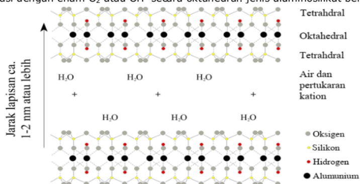
Gambar struktur Montmorilonit ( winaputra 2010)
