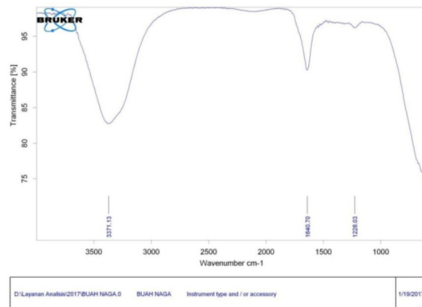
Gambar 4.5 Hasil FTIR.
