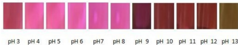
Gambar 4.4 Pengaruh Asam Borak Terhadap Warna Larutan Sesudah Penambahan Buffer
