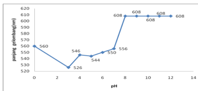
Gambar 4.3. Grafik Hubungan Pengaruh pH dengan Absorbansi
