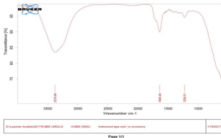
Gambar 4.5. Hasil FTIR
