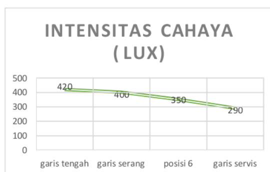
Grafik 2. Intensitas cahaya dari masing-masing titik ukur.
