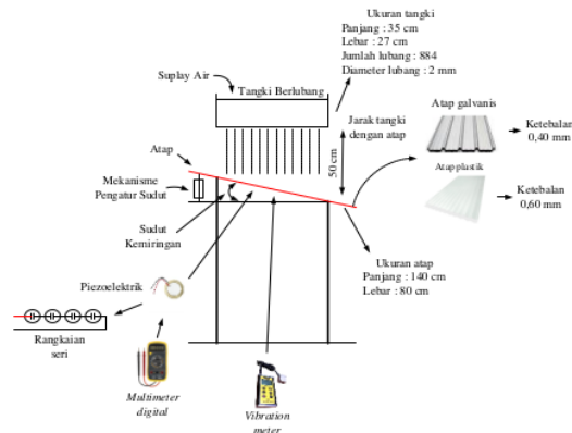
Gambar 2. Skema Alat
