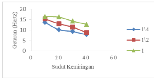
Gambar 3. Grafik pengukuran getaran pada material atap galvalum
