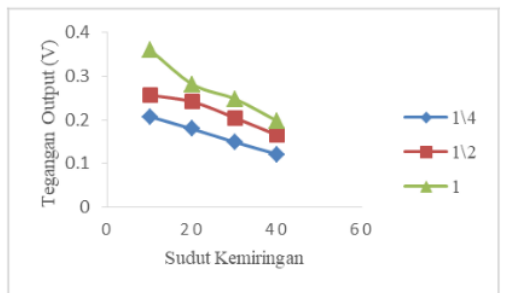
Gambar 6. Grafik pengukuran pada material atap plastik gelombang
