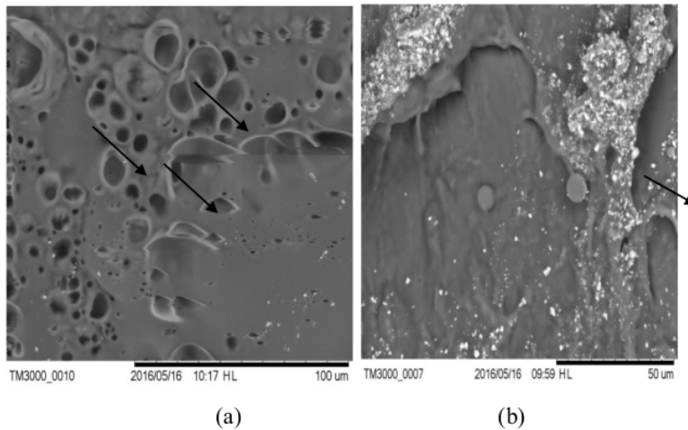
Gambar 4.5 Memperlihatkan hasil fotografi hasil uji SEM dengan perbandingan (a) massa gliserin 6 g, (b) 12 g dengan pembesaran, gambar 400x.
