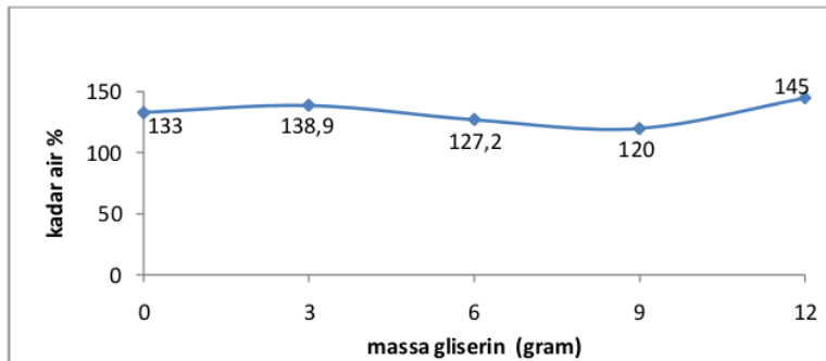
Gambar 4.6. Grafik Uji Kadar Air Edible Film Pektin Dengan variasi massa Gliserin (gram)
