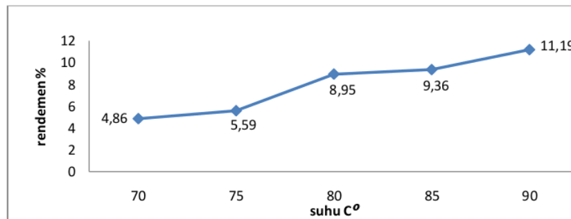
Gambar 4.2. Grafik Pengaruh Suhu Terhadap Hasil Rendemen Pada Ekstraksi Pektin Kulit Pisang Kepok.
