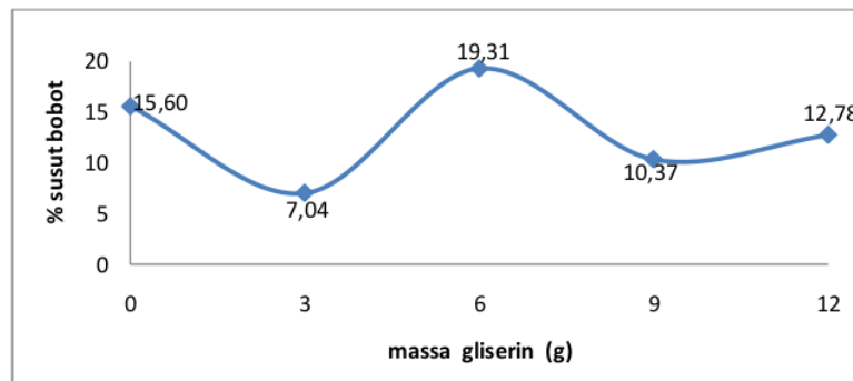
Gambar 4.8 Grafik uji susut bobot dengan lama penyimpanan 3 hari
