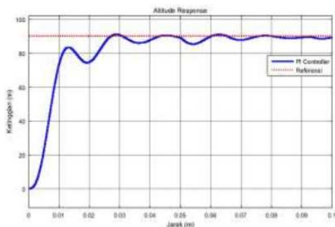
Gambar 11. Respon Motor pada Gerakan Ketinggian 90 m Menggunakan Kontrol PI
