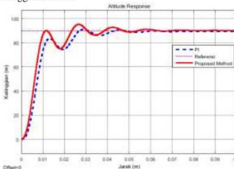
Gambar 16. Respon Motor pada Gerakan Ketinggian 90 m Menggunakan Kontrol PID
