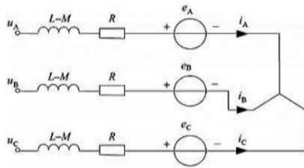
Gambar 5. Rangkaian Ekuivalen Motor BLDC [12]
