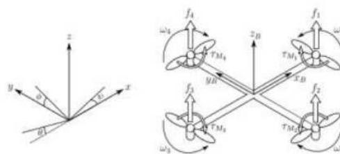
Gambar 3. Kerangka Inersia Quadcopter [10].
